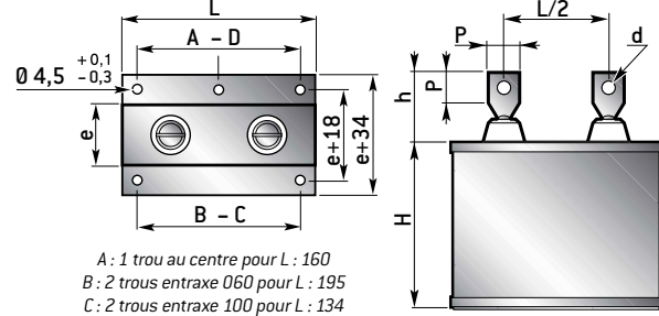
PLP 80 with mounting bracket / avec fixation
