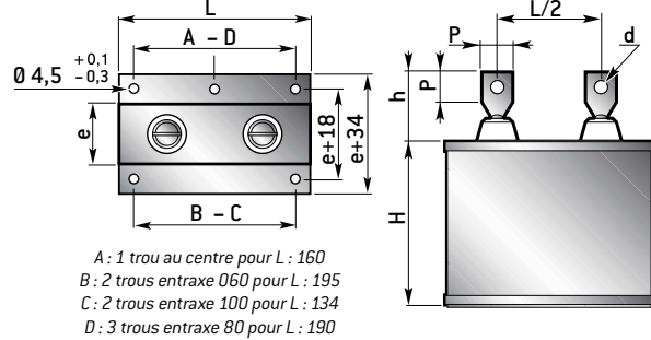
PLP 80 with mounting bracket / avec fixation
