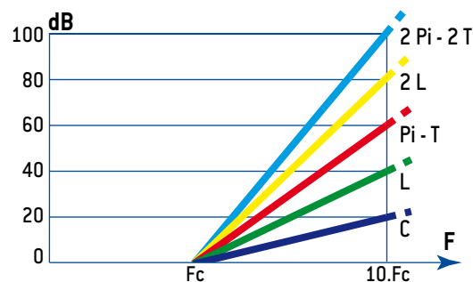
Attenuation by structure / Atténuation par structure
