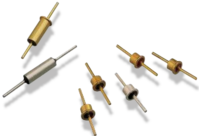
Filtres miniatures (Ø 3 mm)
