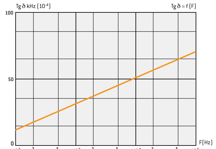
Dissipation factor change versus frequency / Évolution de la tangente de l'angle de pertes en fonction de la fréquence
