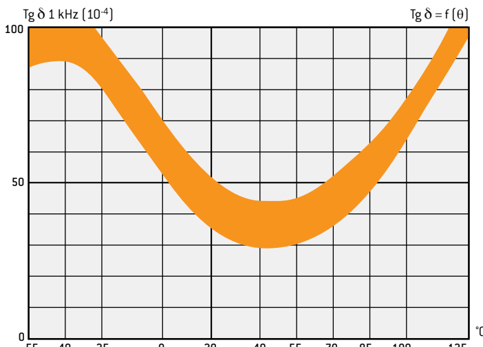
Dissipation factor change versus temperature / Évolution de la tangente de l'angle de pertes en fonction de la température
