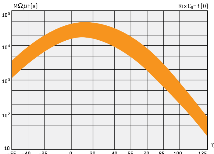
Insulation resistance change versus temperature / Évolution de la résistance d'isolement en fonction de la température
