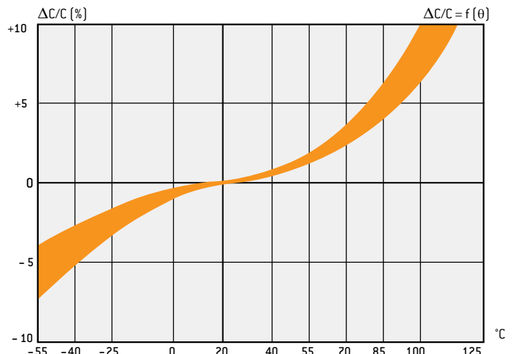
Relative capacitance variation versus temperature / Variation relative de la capacité en fonction de la température
