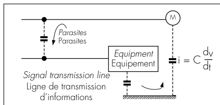
Exemple de couplage capacitif.
