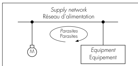
Exemple de couplage résistif (galvanique).
